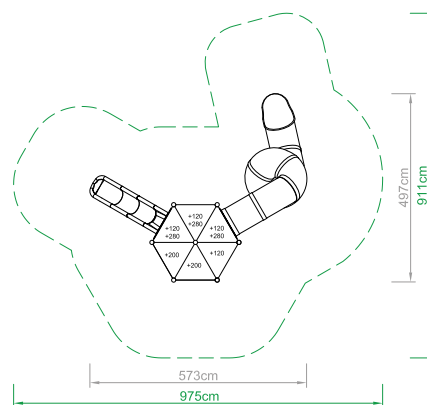
Planta en área de seguridad
