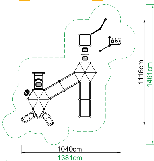
Planta en área de seguridad
