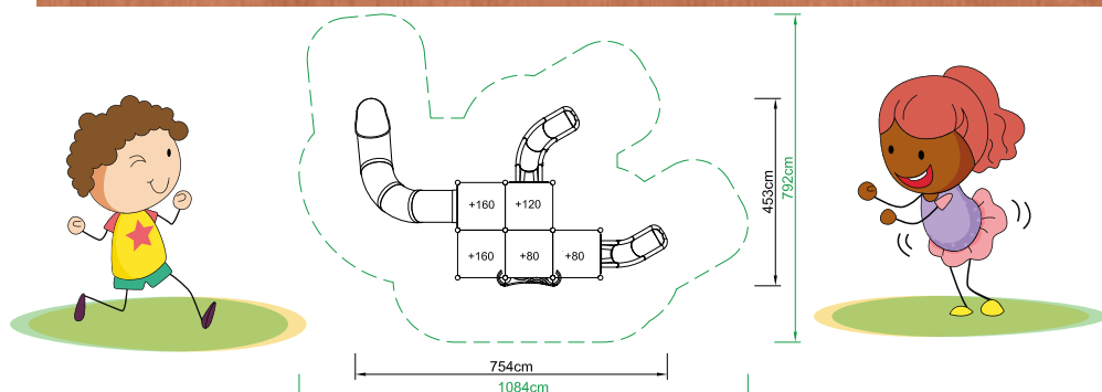
Planta en área de seguridad
