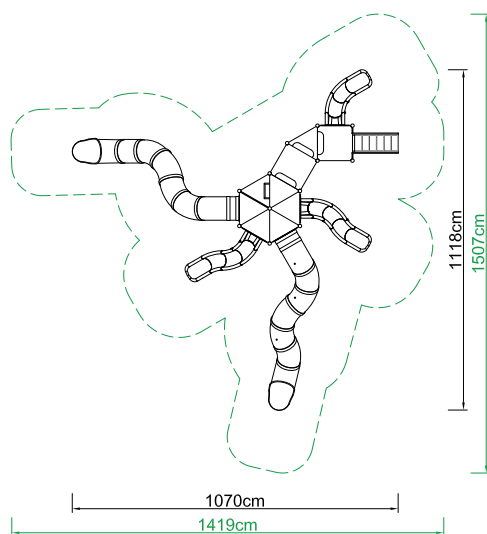
Planta en área de seguridad
