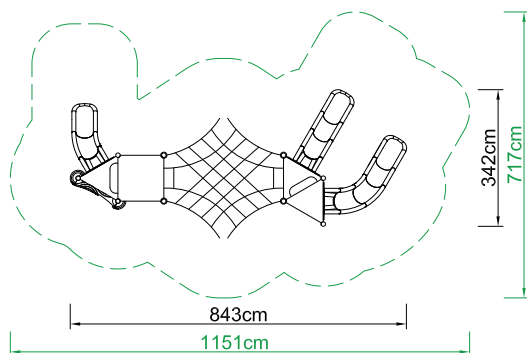
Planta en área de seguridad
