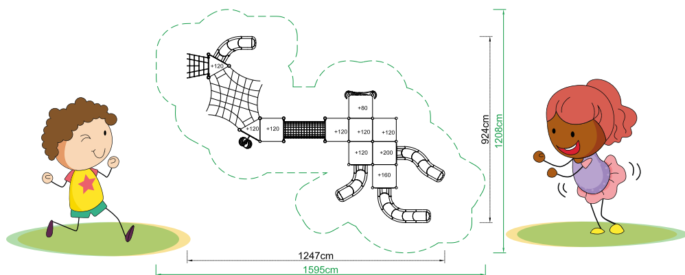
Planta en área de seguridad
