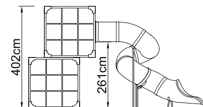
Medidas alzado
