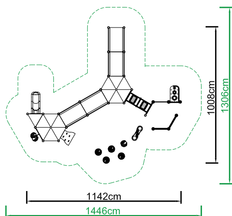
Planta en área de seguridad
