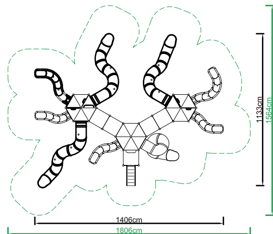
Planta en área de seguridad
