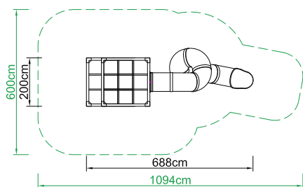
Planta en área de seguridad
