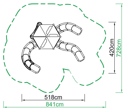
Planta en área de seguridad
