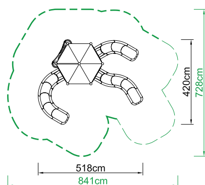
Planta en área de seguridad
